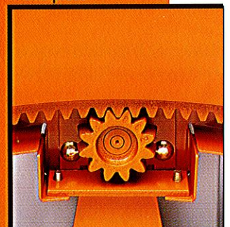
Einstellbares Zahnspiel. Battement réglable. Gap between pinion and gear ring is adjustable.
