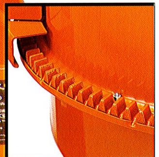
Einteiliger Spezialguß-Zahnkranz. Couronne en fonte spéciale. Special cast iron gear ring, made in one piece
